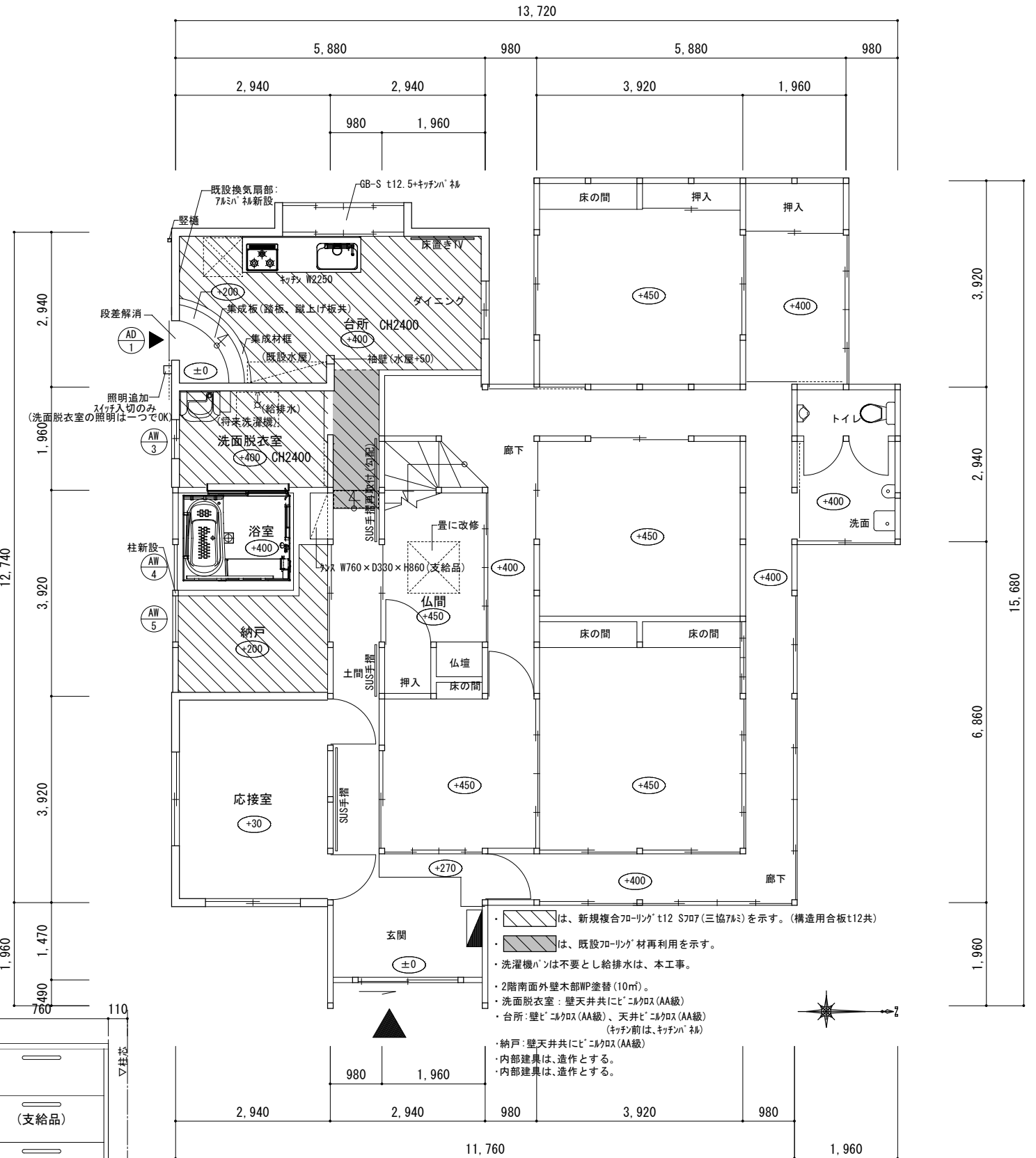
(改修後) 1階平面図 S=1/100
