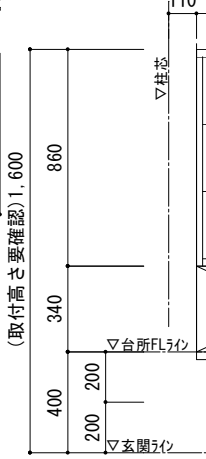
階段断面
